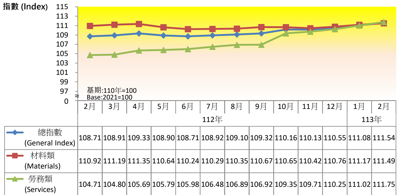
圖3 新北市營造工程物價指數趨勢圖 Trends of Construction Cost Indices in New Taipei City
